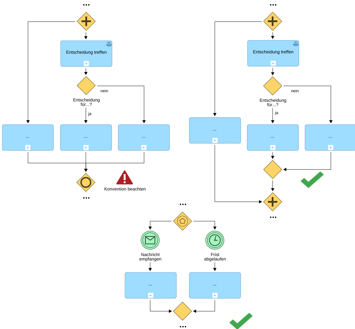
Abbildung 15 Verzweigung und Zusammenführung durch denselben Gateway-Typ
