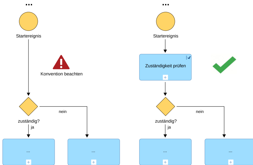
Abbildung 16 Prüf-Aktivität vor Verzweigung
