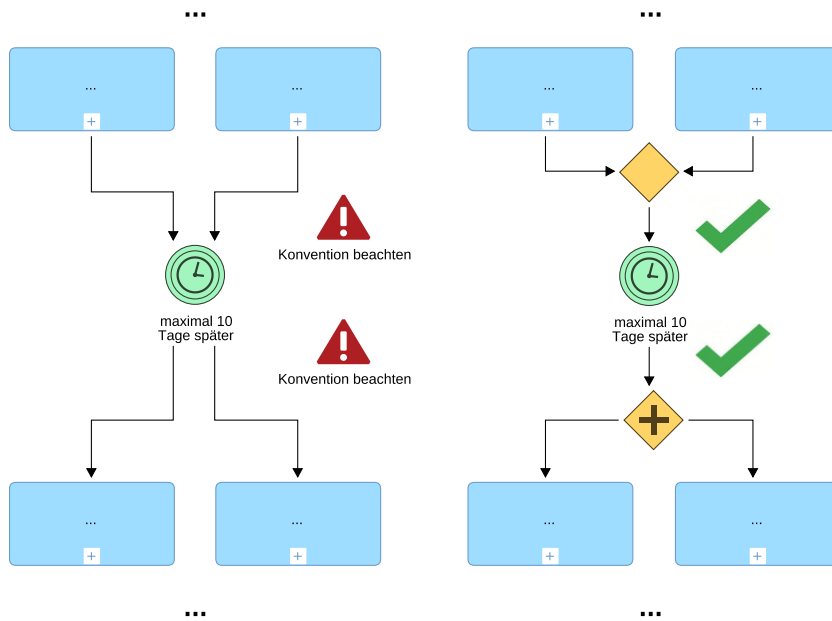
Abbildung 18 Zwischenereignis mit ein- und ausgehendem Kontrollfluss
