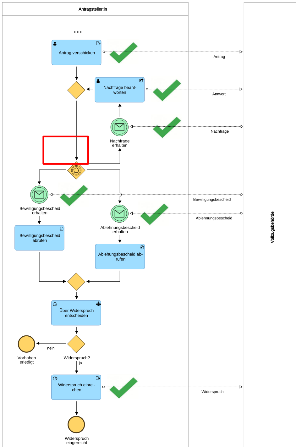
Abbildung 20 Nachrichten-Zwischenereignis nach ereignisbasierter Verzweigung
