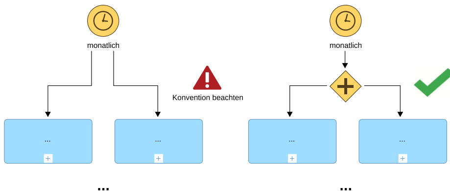
Abbildung 17 Startereignis - ausgehende Kontrollflüsse
