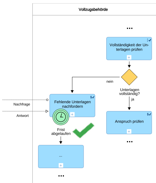
Abbildung 19 Randereignis (angeheftetes Zwischenereignis)
