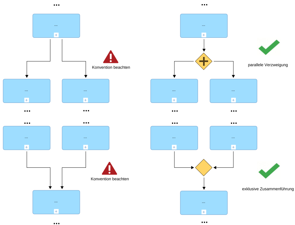
Abbildung 13 Gateway - Verzweigung und Zusammenführung von Kontrollflüssen
